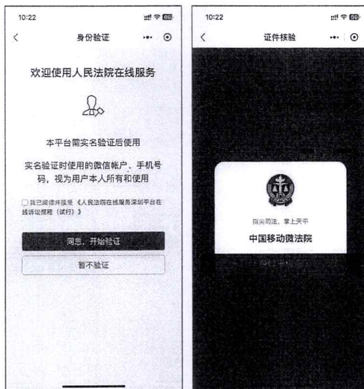
图 1.1-2 证件核验
