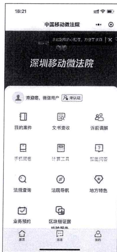
图 1.1-1 首页
