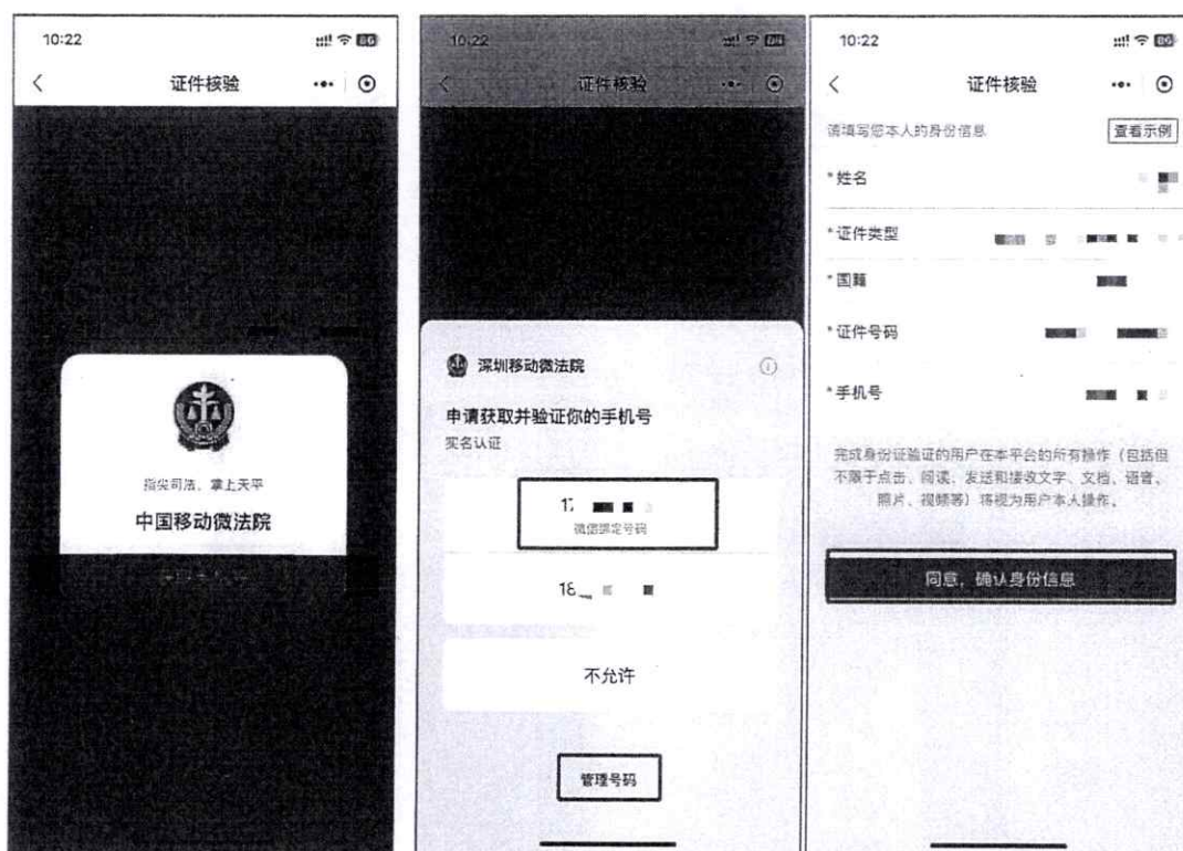
图 1.1-3 获取手机号
